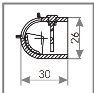
PRZEKRÓJ OZ 100
