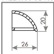
PRZEKRÓJ OZ 300
