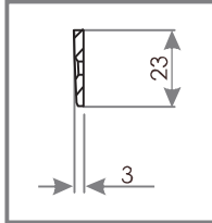
PRZEKRÓJ OZ 300
