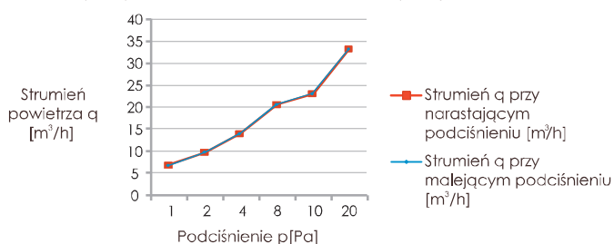
Wykres 6. Zależność strumienia powietrza q [m 3 /h] przepływającego przez nawiewnik VT 401 od panującego podciśnienia p [Pa]
