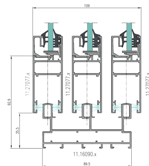
Wersja 3-szynowa.
