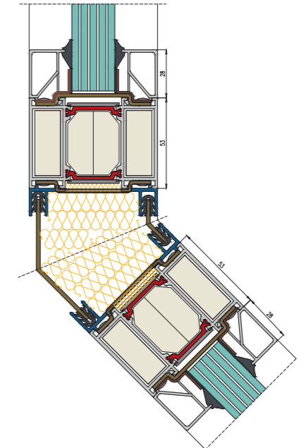
Połączenie narożne 135°.
