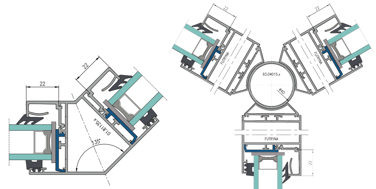
Profil narożny 135°.
