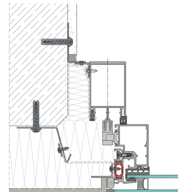
Połączenie słupa ze ścianą budynku.
