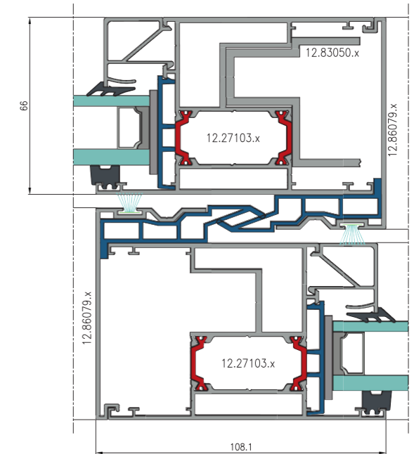
Zejście skrzydeł.
