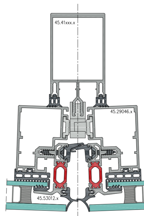
Przekrój przez słup.
