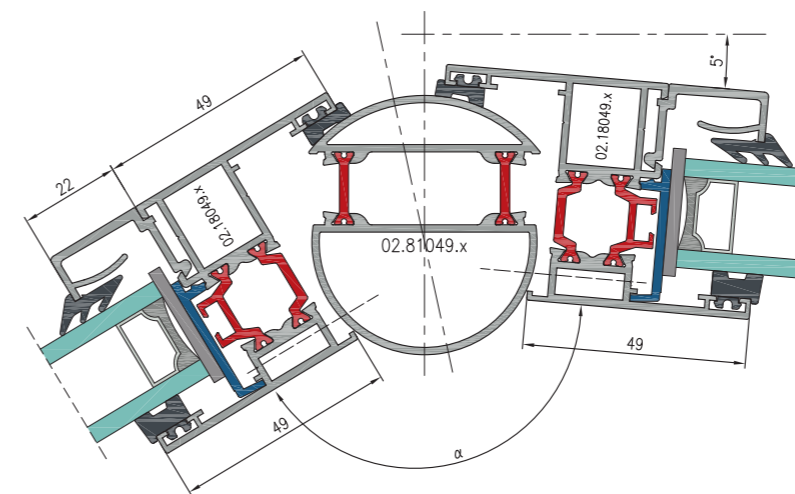
Rozwiązanie kątowe 90 - 170°.
