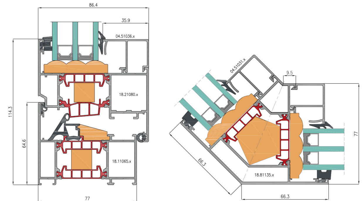
Przekrój przez skrzydło i ościeżnicę.
