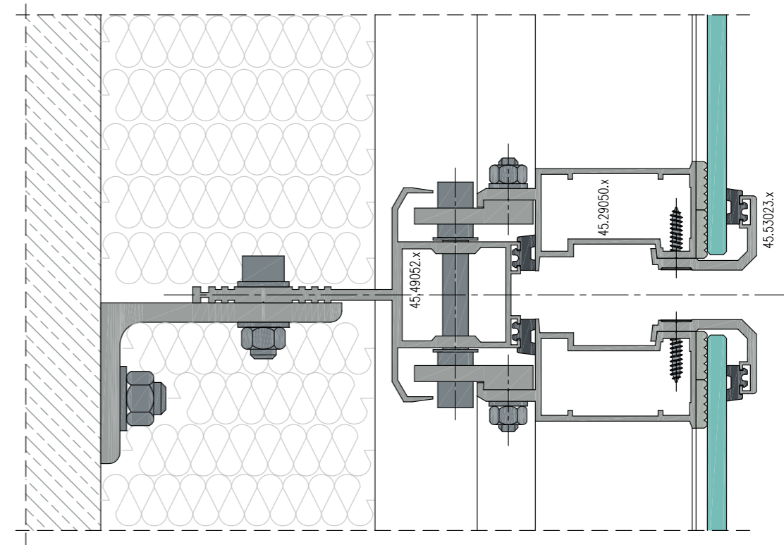
Przekrój przez słup.
