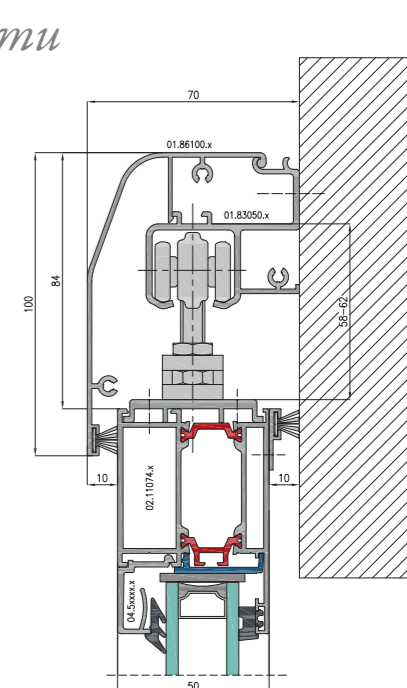
Drzwi podwieszane.
