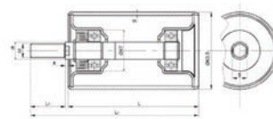
Rolki kierunkowe
