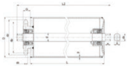
Rolki łańcuchowe
