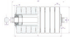
Krążniki pierścieniowe
