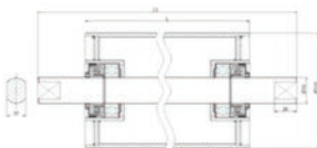
Krążniki odciskowe
