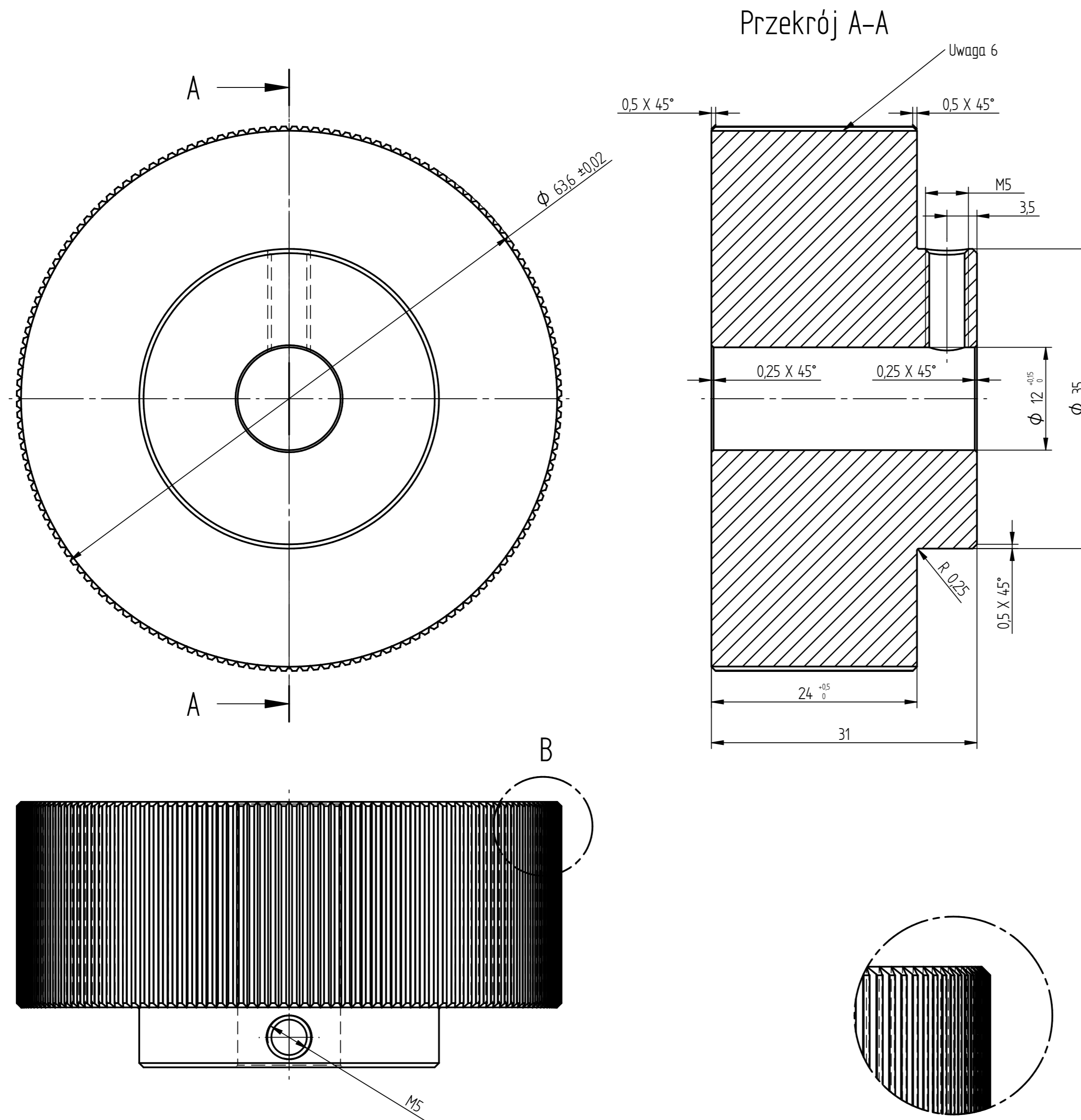
Szczegół B
