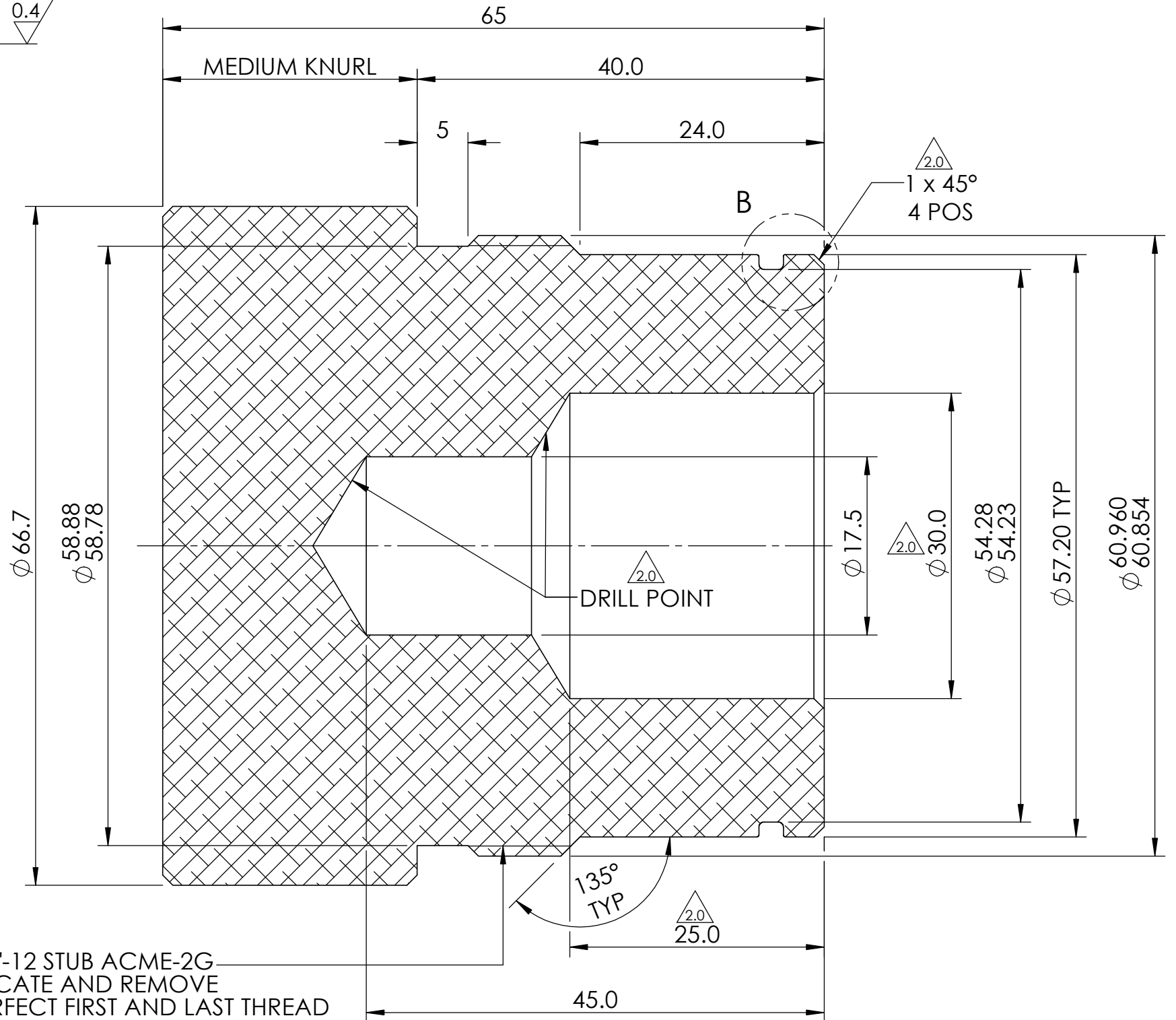
SECTION A-A
