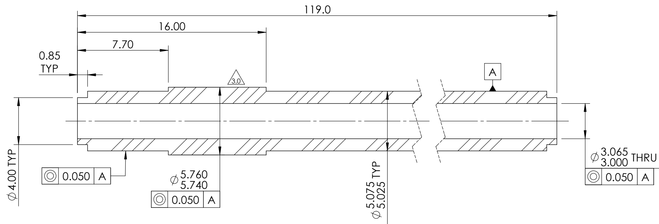
SECTION A-A
