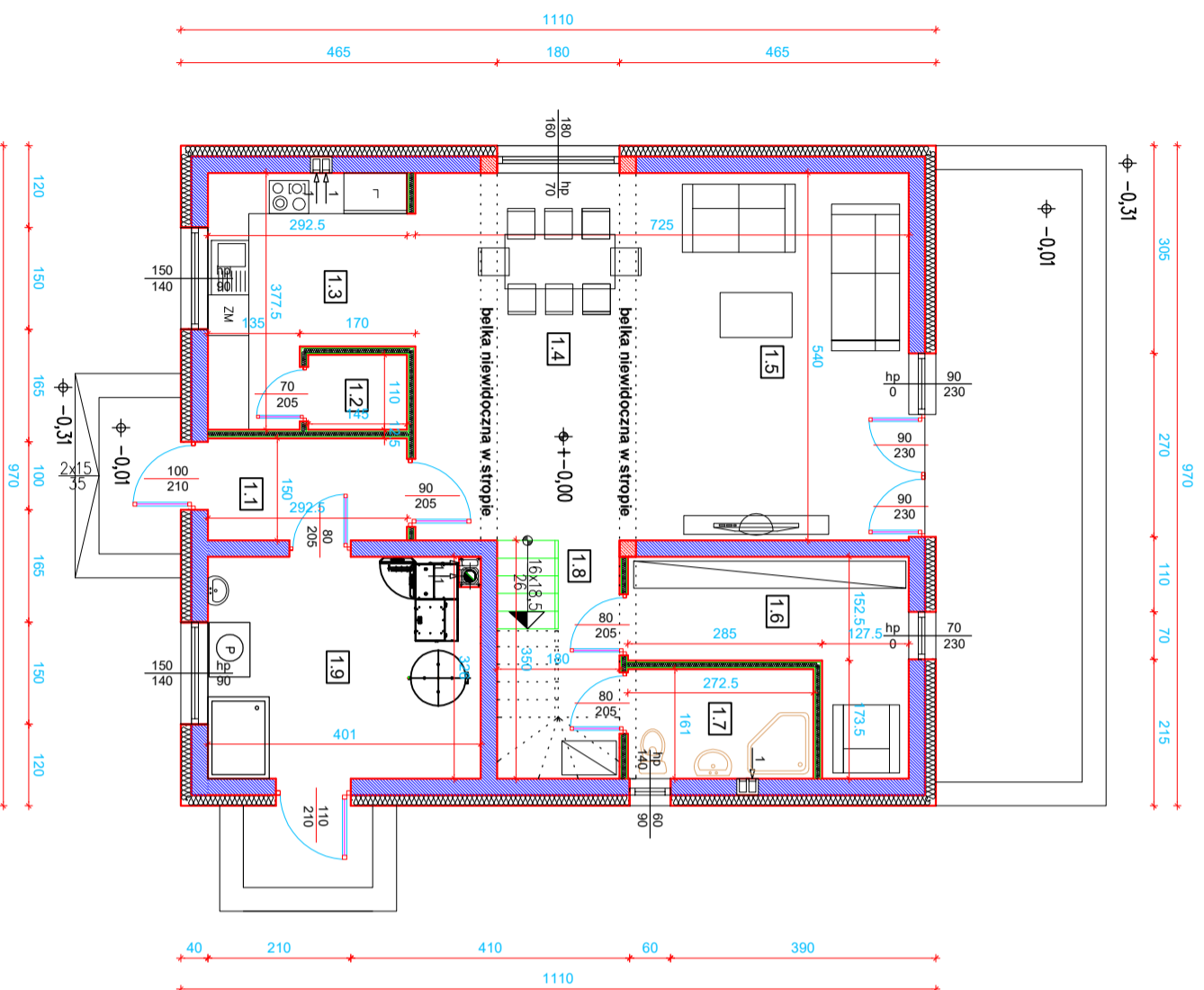
RZUT PARTERU
