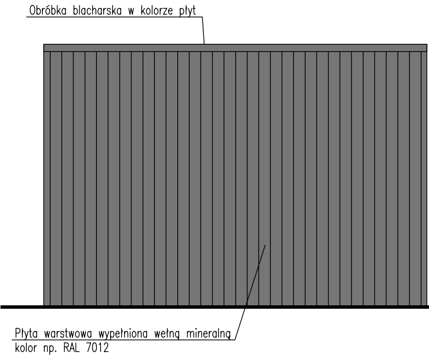
WIDOK ŚCIANY W OSI 2
