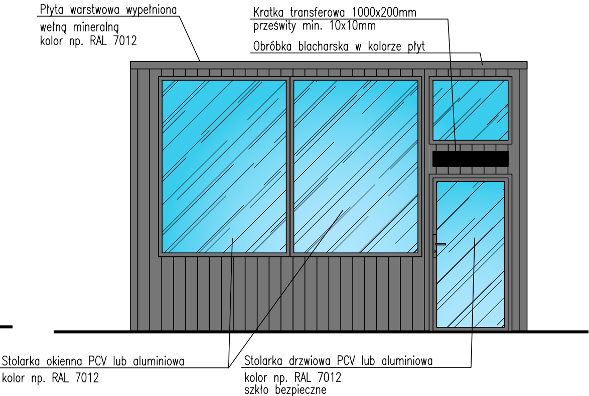
WIDOK ŚCIANY W OSI B
