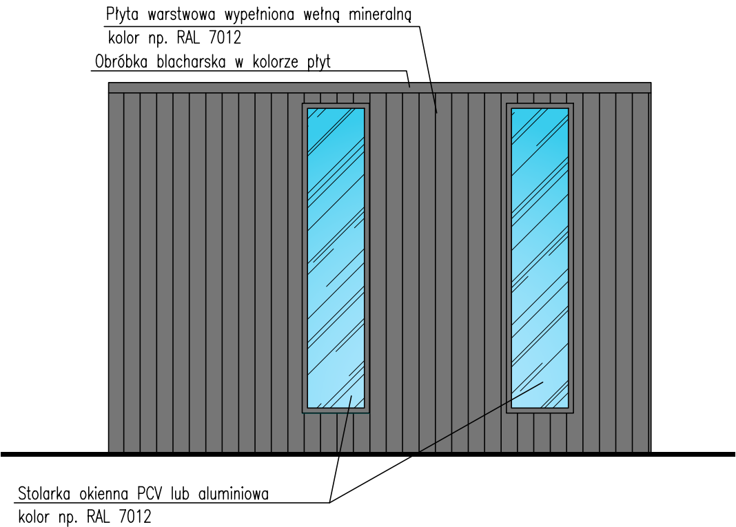
WIDOK ŚCIANY W OSI 1
