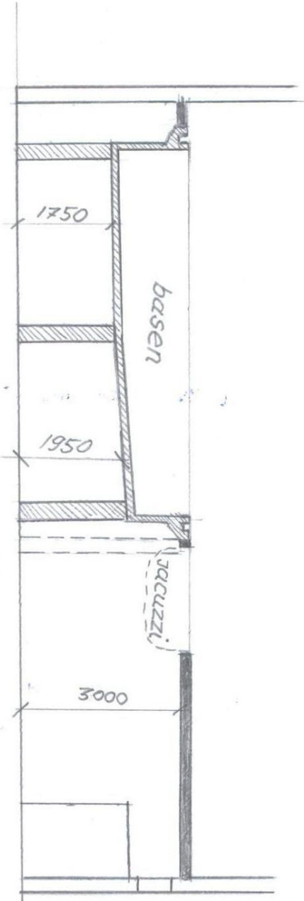
Przekrój AA
