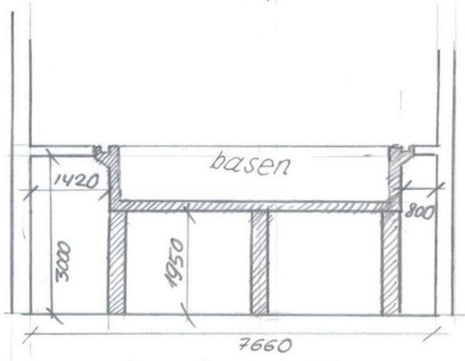
Przekrój BB
