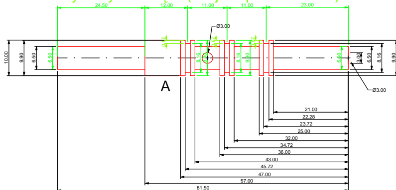
Wymiarowanie podstawowe
