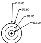
Rzut z tyłu (od strony otworu 3mm)
