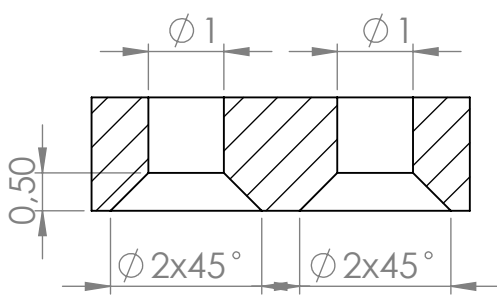
PRZEKRÓJ A-A
